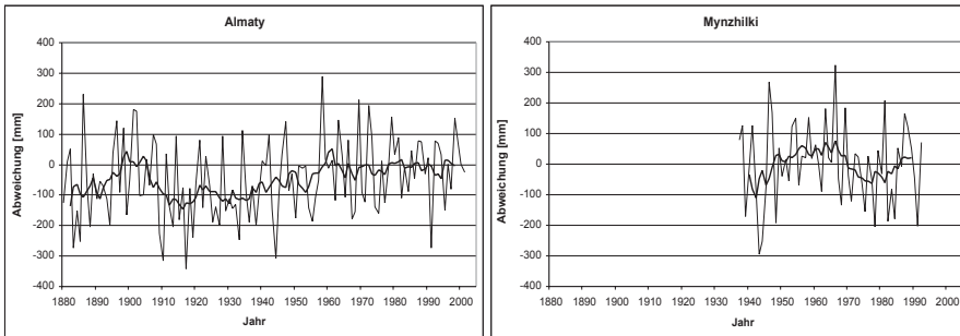
Abb. 5: Zeitreihen der Niederschlagsabweichung ausgewählter Klimastationen vom Durchschnitt der Klimanormalperiode 1961-90, dicke Linie: 7-jähriges gleitendes Mittel
