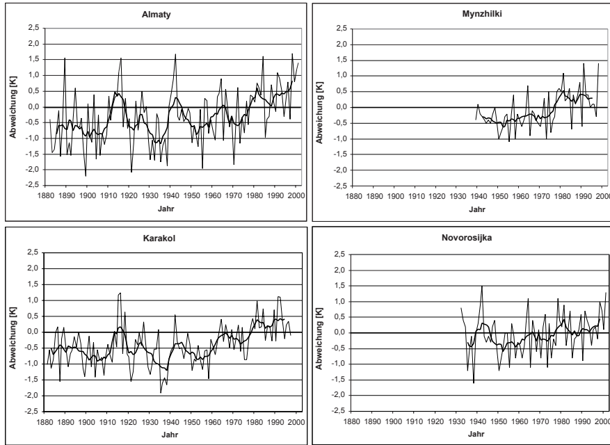
Abb. 4: Zeitreihen der Temperaturabweichung ausgewählter Klimastationen vom Durchschnitt der Klimanormalperiode 1961-90, dicke Linie: 7-jähriges gleitendes Mittel
