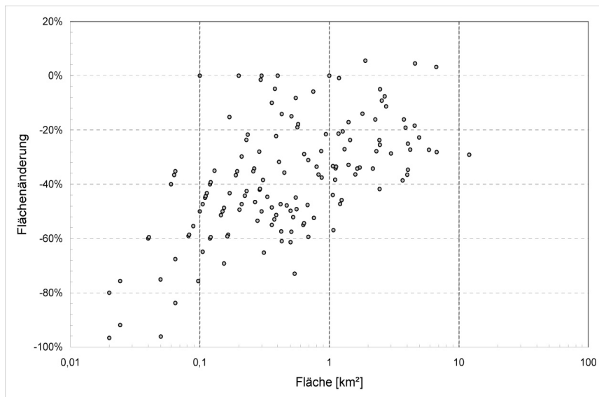
Abb. 8: Änderung der Gletscherfläche im Verhältnis zur Gletschergröße; man beachte die logarithmische Skala der Abszisse
