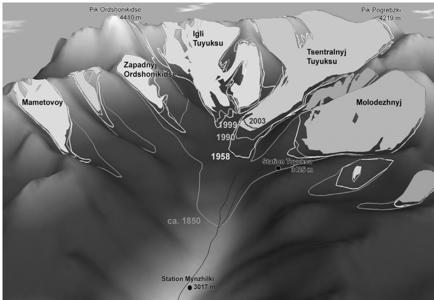
Abb. 6: Gletscherschwund im Malaja Almatinka Tal
