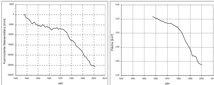
Abb. 7: Links: Kumulierte Massenbilanz des Tujuksu-Gletschers; 1937-56 modelliert aus Klimadaten, ab 1957 gemessene Daten; rechts: Flächenveränderung Quellen: DYURGEROV ET AL. 1996, WGMS
