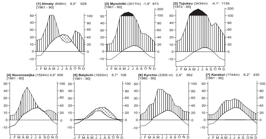
Abb. 2: Ausgewählte Klimadiagramme; zur Lage vgl. Abb. 1
